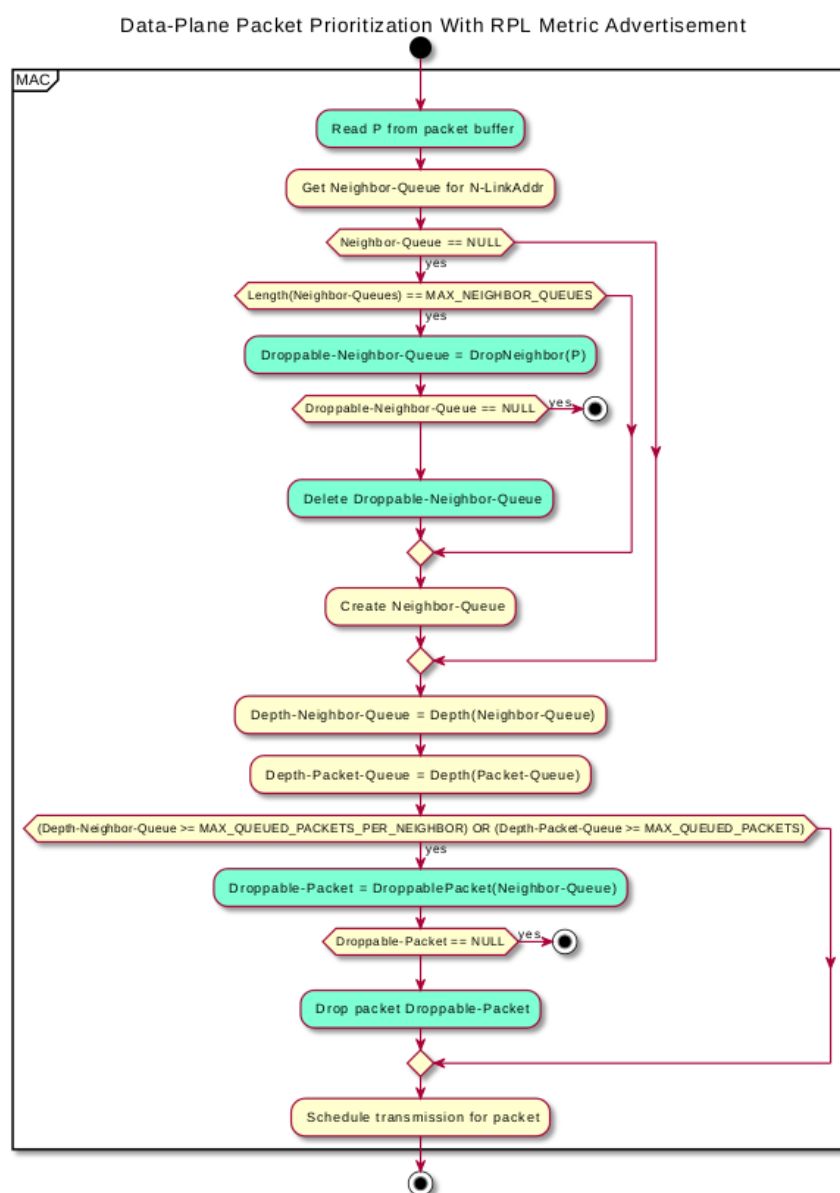
Fig. 5: MAC Layer
