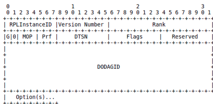
Fig. 2: DIO - Message format [10]
